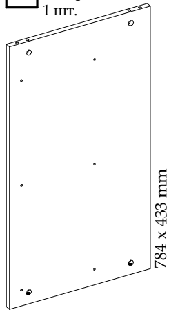
2 Боковина центральна ліва 1 шт.
