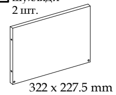
8 Задня стінка шухляди 2 шт.
