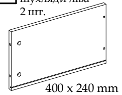
8 Задня стінка шухляди 2 шт.
