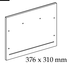
16 Фронт шухляди 2 шт.
