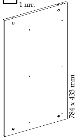
3 Боковина центральна права 1 шт.
