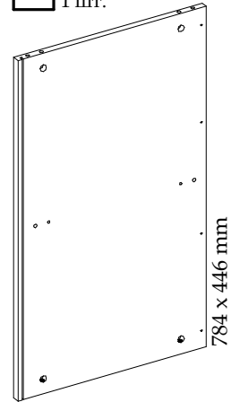
4 Боковина права 1 шт.
